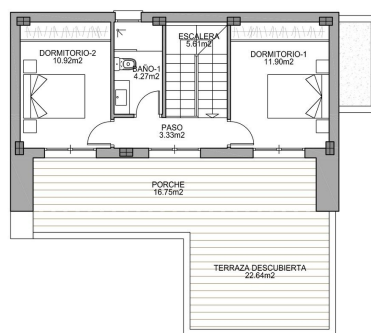
PLANTA PRIMERA
