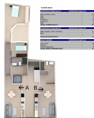
Planta Baja. Estudio B y Vivienda A
