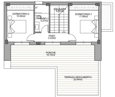
PLANTA PRIMERA
